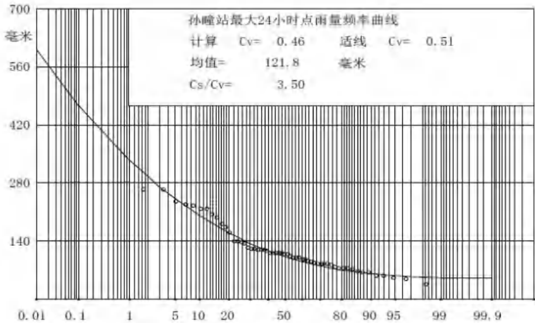
图 2.1-1 孙疃站最大 24 小时降雨频率曲线（1967～2021 年）
