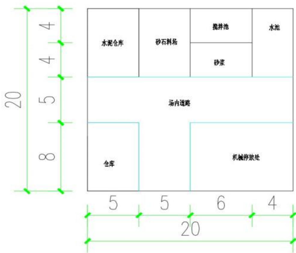
图 2-1 施工平面布置图
