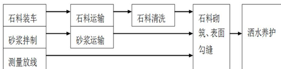
图 2-3 砌石施工工艺流程图
